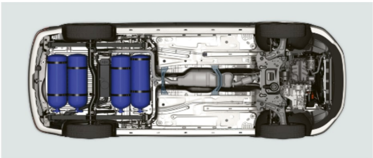
Die Unterflur-Gasstahltanks – vier beim Caddy, fünf beim Caddy Maxi – sind so verbaut, dass es keine Abstriche bei Laderaum und Ladekantenhöhe gibt.
