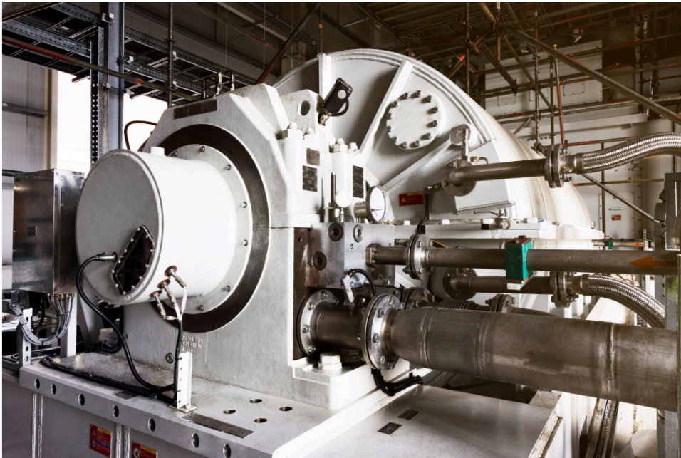
Roterande stabilisatorer som används i länder med mycket vindkraft och liten svängmassa. Här Irland, man även i Spanien och Australien.
